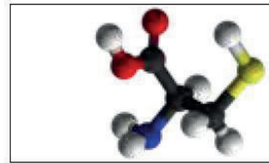
Cysteinsyre
